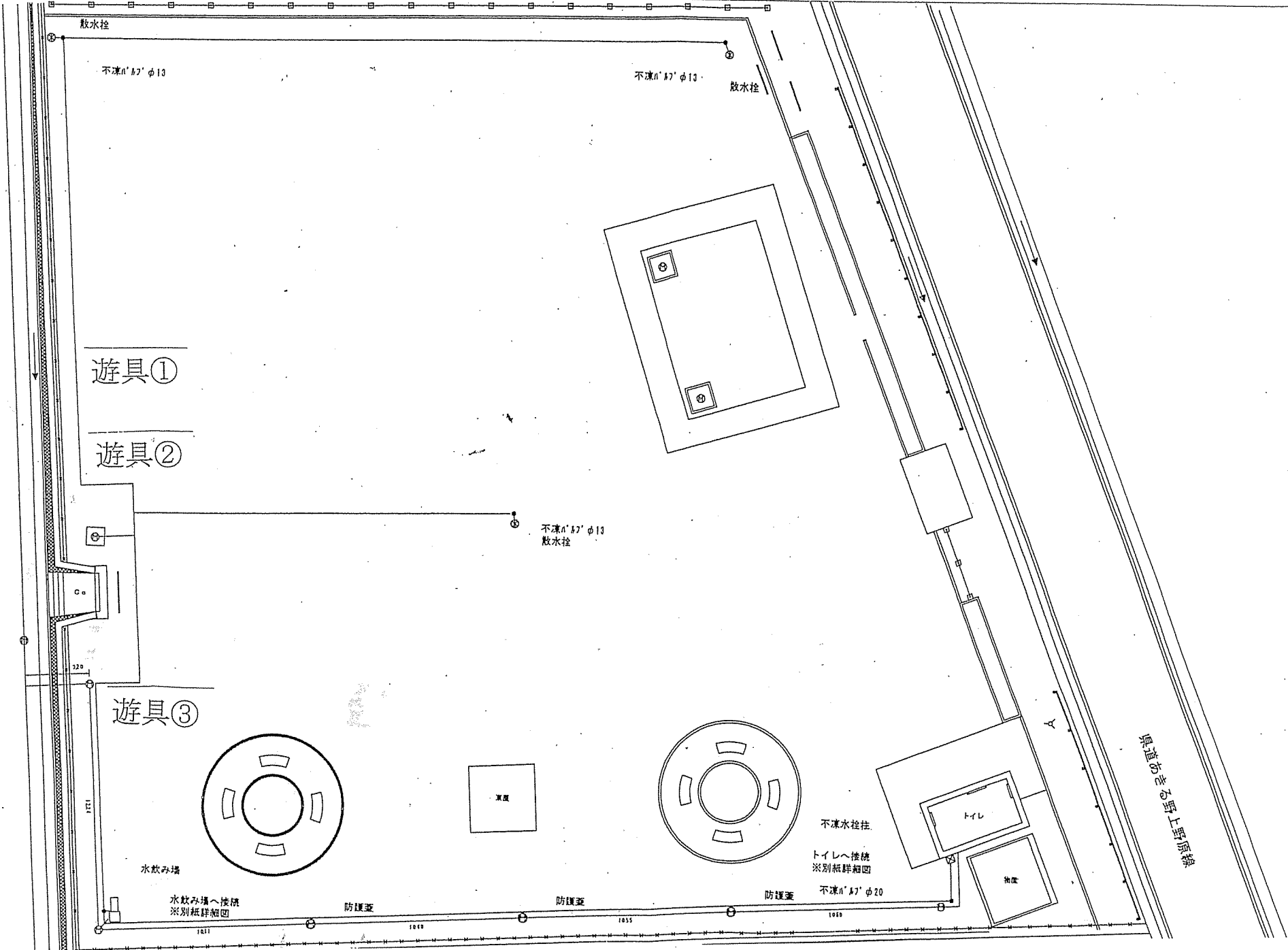
上野原市中央防災公園遊具設置工事配置図
